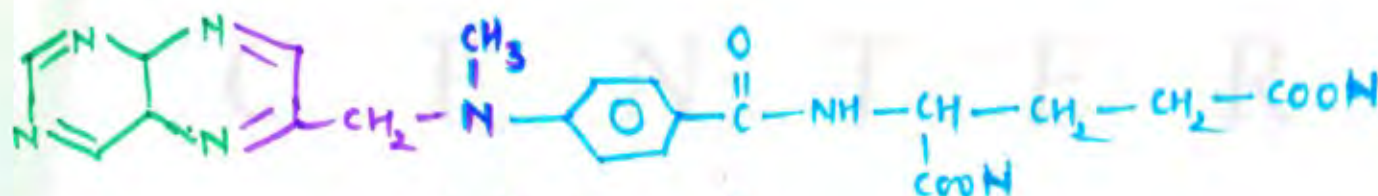
Methotrexate
